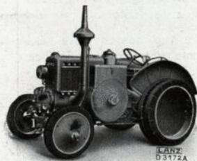
30 PS Verkehrs-Bulldog mit Auspuff nach oben oder unten
