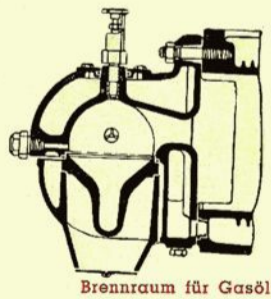
Brennraum für Gasöl
