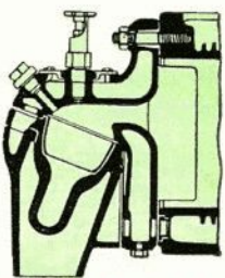
Brennraum für Spiritus
